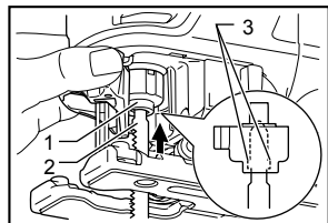
1. Porte-lame 2. Lame de scie sauteuse 3. Saillies
